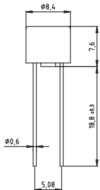
Abmessungen Dimensions
