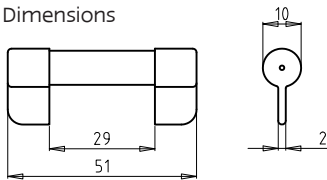
Abmessungen Dimensions
