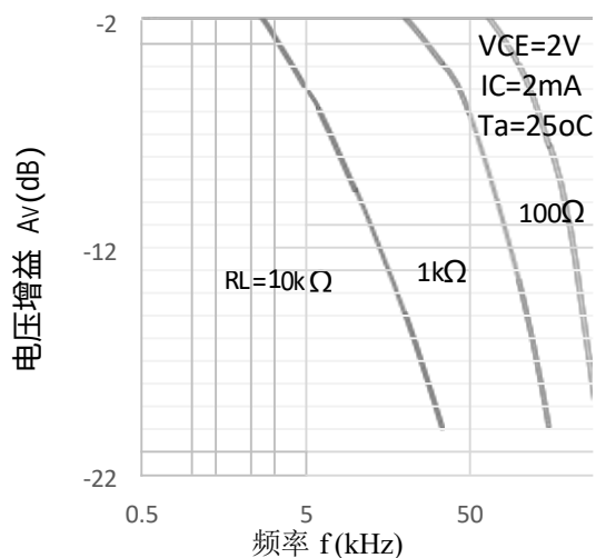
频率响应曲线图
