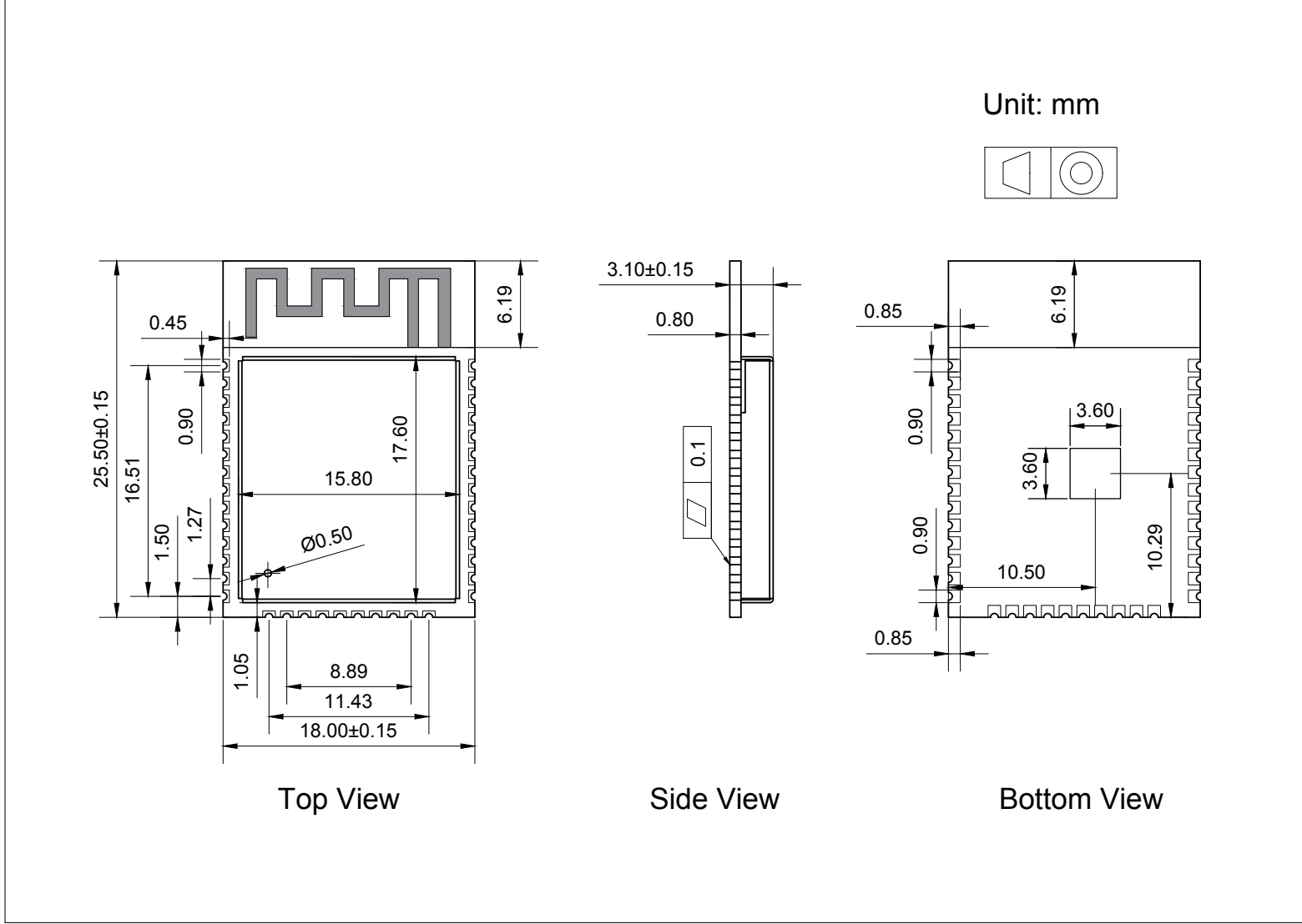
图 5: ESP32-SOLO-1 尺寸
