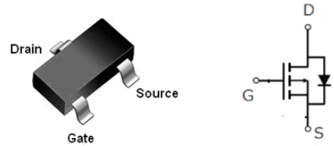
SOT23
