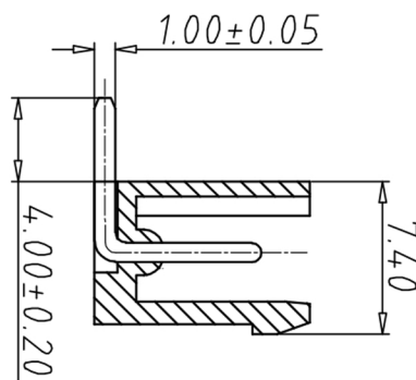
剖视图 A-A
