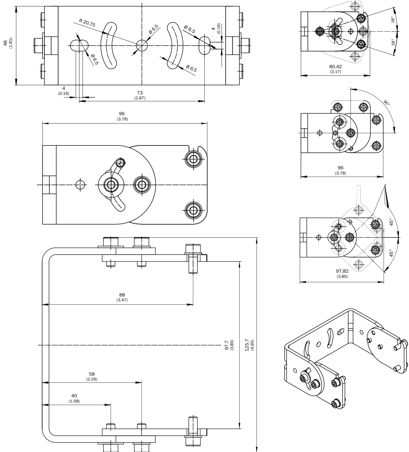
尺寸图 (尺寸单位: mm)
