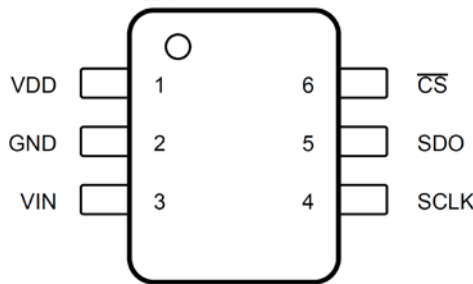
引脚图
