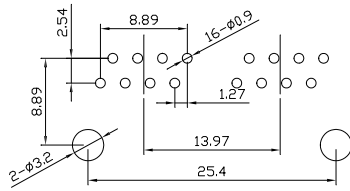
P.C.B参考图
