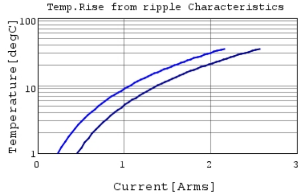
GRM155R61A105KE01 Temp.rise — 500kHz —
