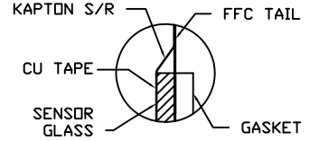
SECTION A-A SCALE: 8/1
