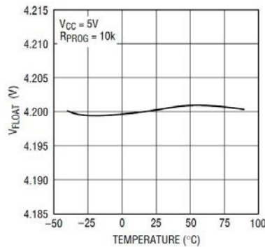
浮充电压 vs 温度
