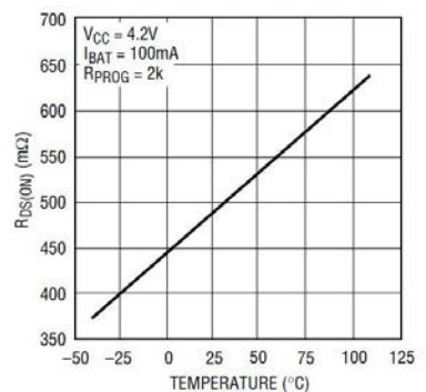
功率 MOS 开态电阻 vs 温度
