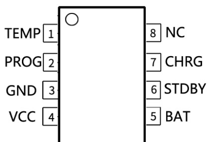
ESOP-8
