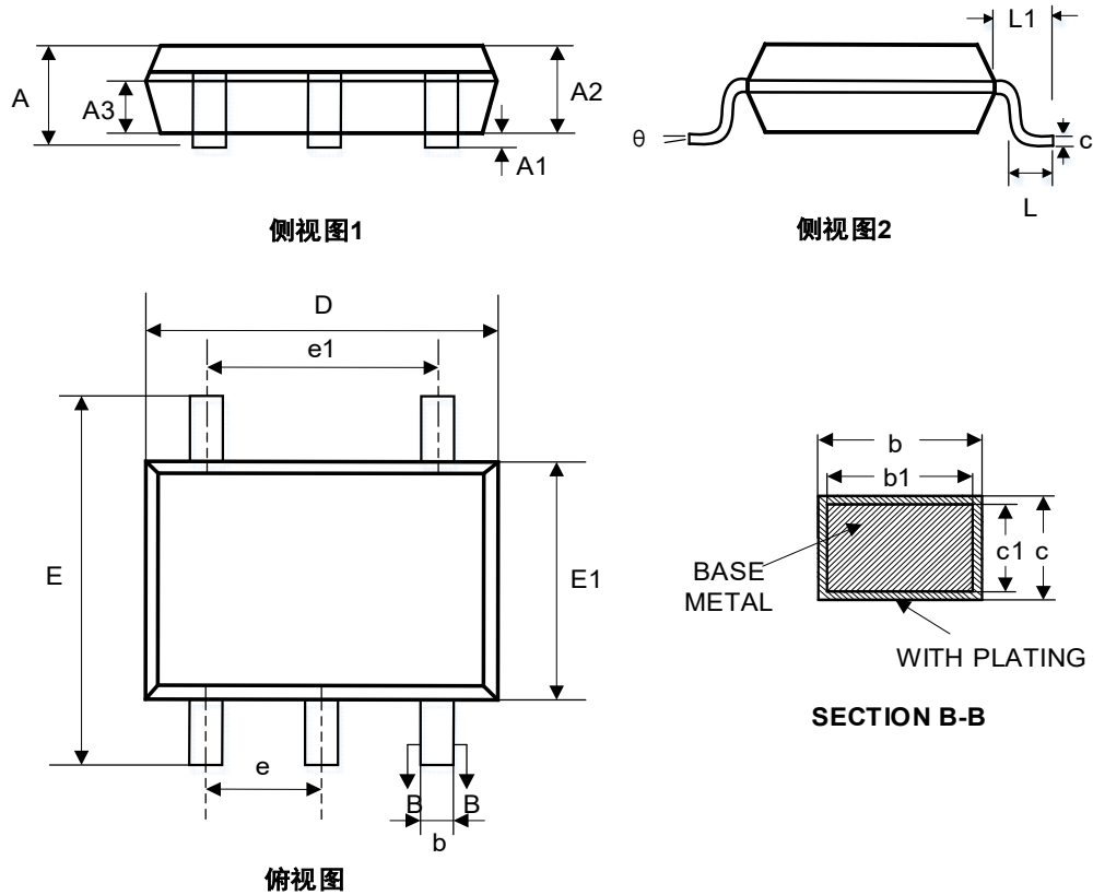
图12.2 IBSP3032 SOT23-5封装尺寸
