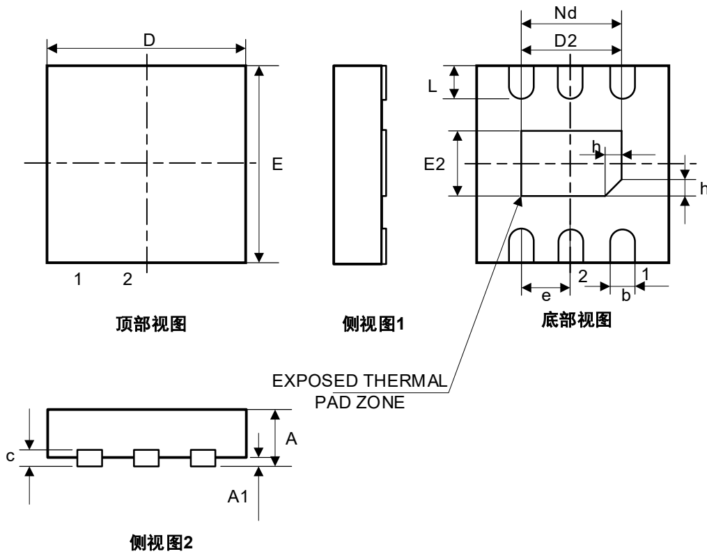
图12.1 IBSP3032 DFN-6(2mm×2mm)封装尺寸
