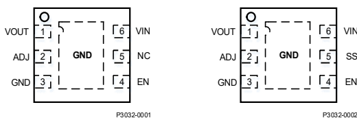
图4.1 DFN-6封装 注1 (2mm×2mm×0.73mm)
