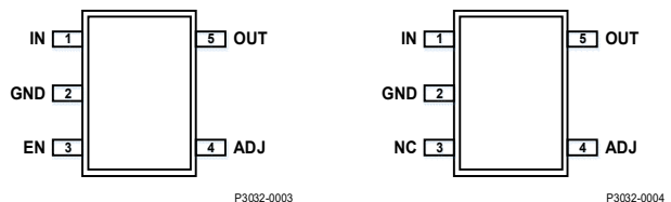
图4.2 SOT23-5封装 注2 (2.92mm×2.8mm×1.1mm)
