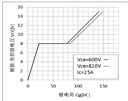
图 6 栅电荷特性
