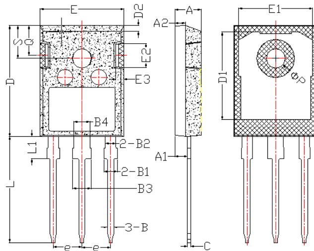
外形图:
