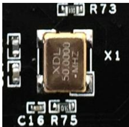
图 4.2 50M 有源晶振实物图
