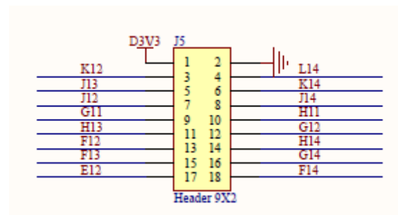
图 14.1 摄像头接口原理图
