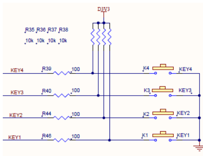
图 13.1 4 个用户按键原理图
