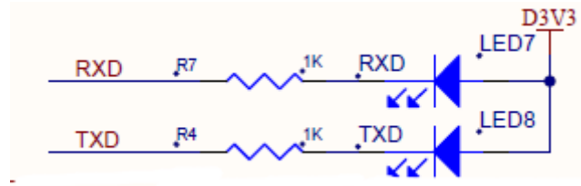
图 9.3 USB 转串口信号指示灯
