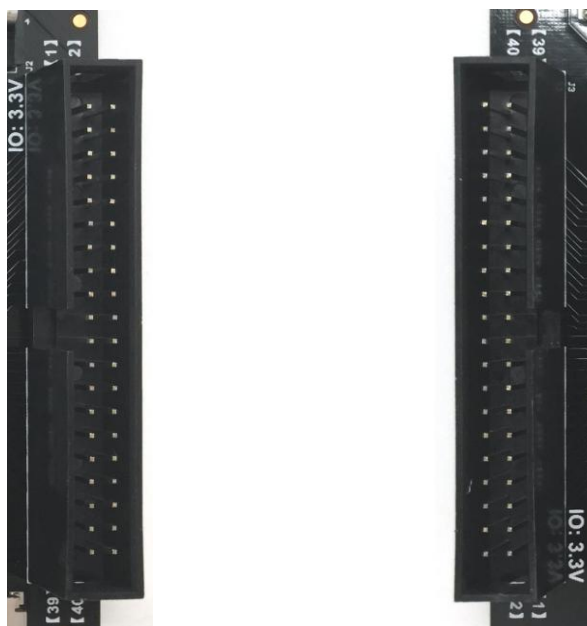
图 17.3 J2, J3 扩展口实物图
