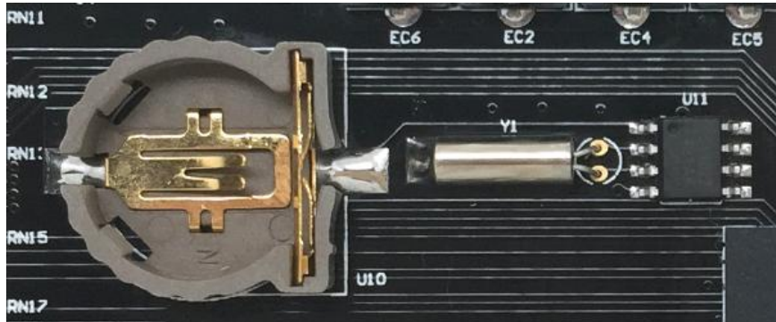
图 8.2 DS1302 实物图
