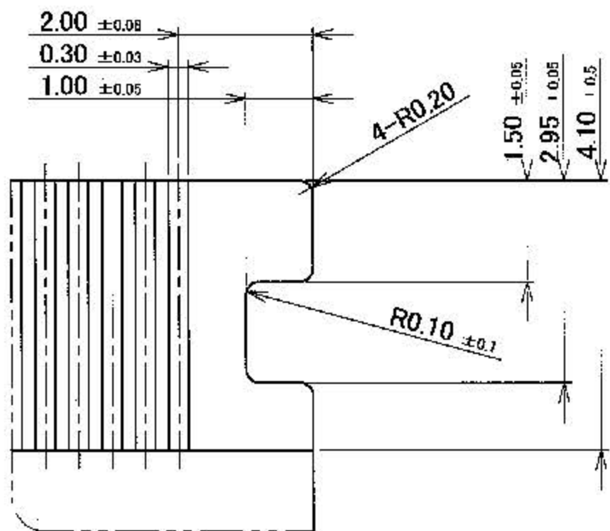
DETAIL Y (S=10/1)
