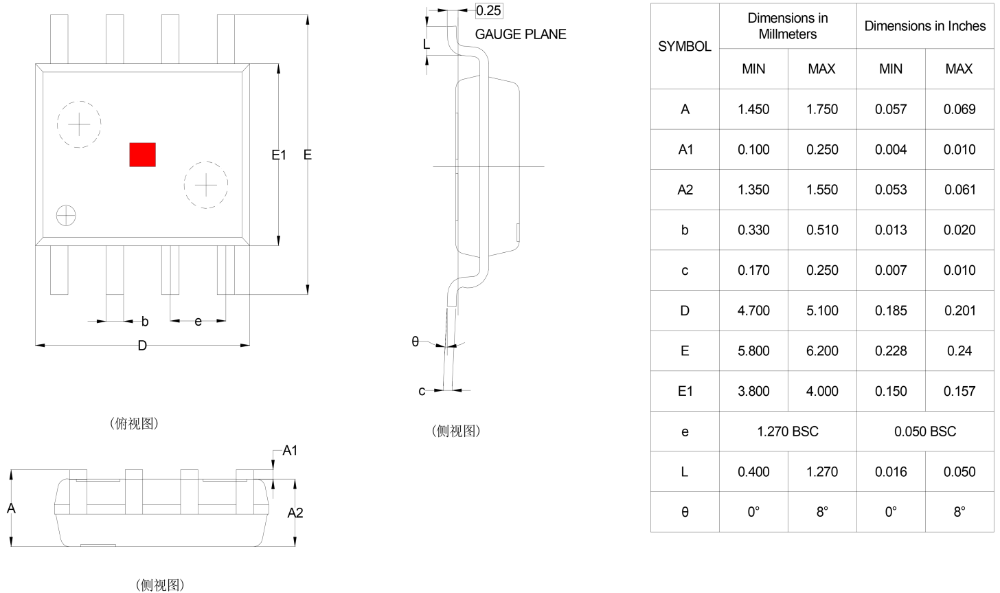
图示：SOP8 封装外形（单位：毫米）
