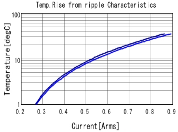
GJM1555C1H2R0WB01 Temp. rise ■ 2GHz ■ 3GHz
