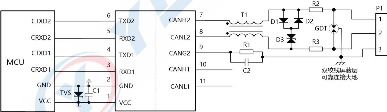
图 2. EMC 推荐电路
