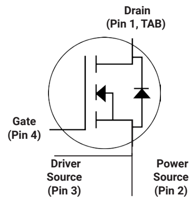
TO-247-4
