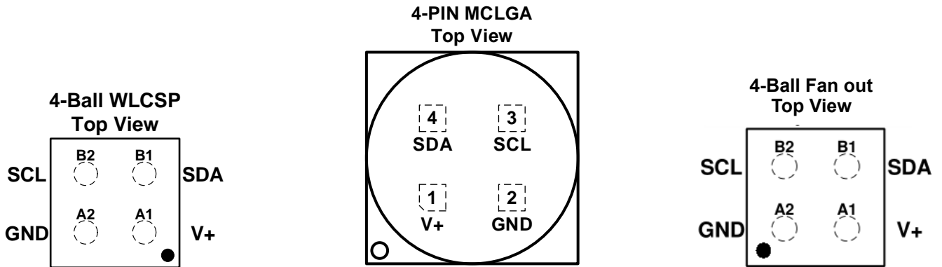
引脚功能
