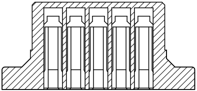
SEC:A-A
