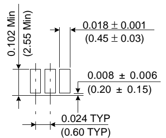
Detail Y
