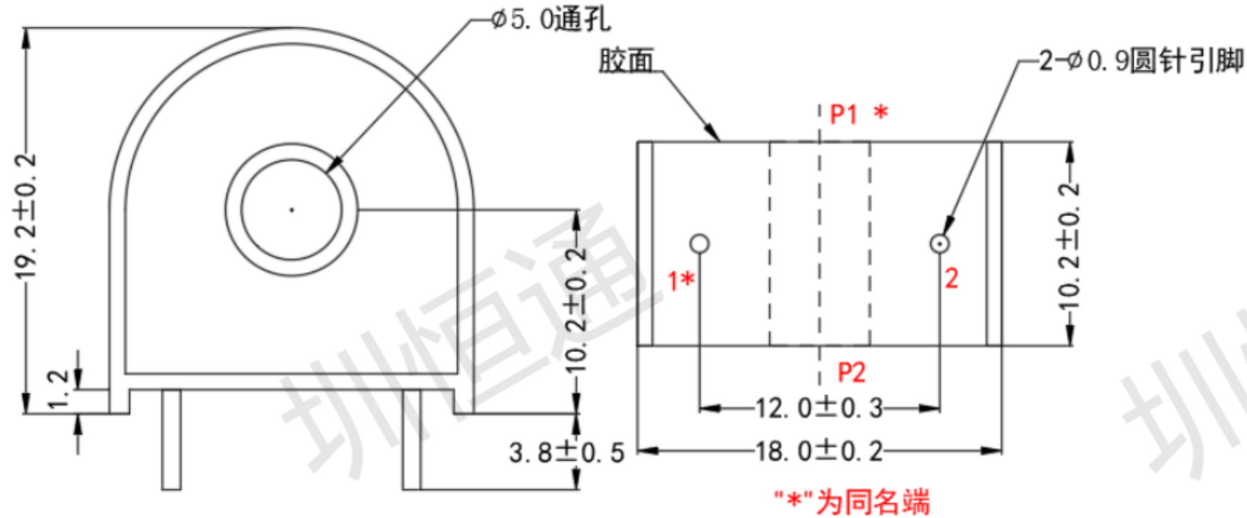
主视图
