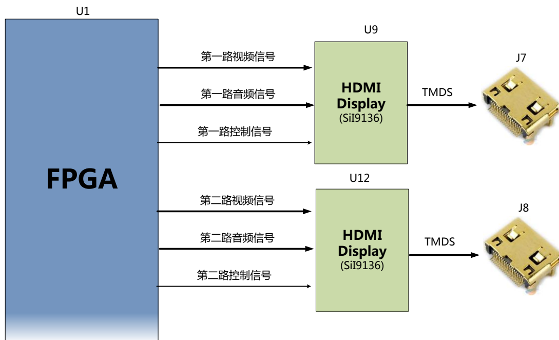
图 3-3-1 HDMI 输出接口设计原理图
