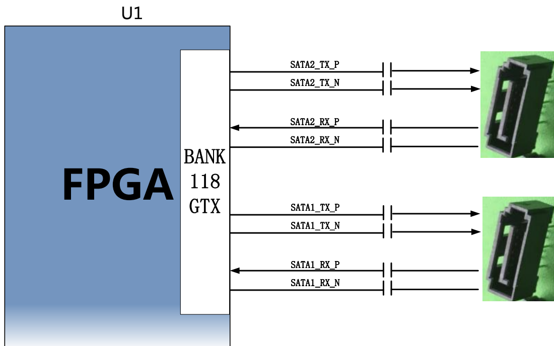
图 3-5-1 SATA 接口设计示意图
