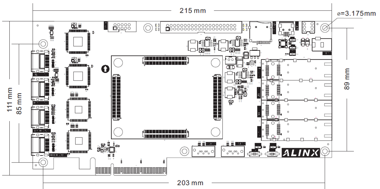
图 3-12-1 正面图 ( Top View )
