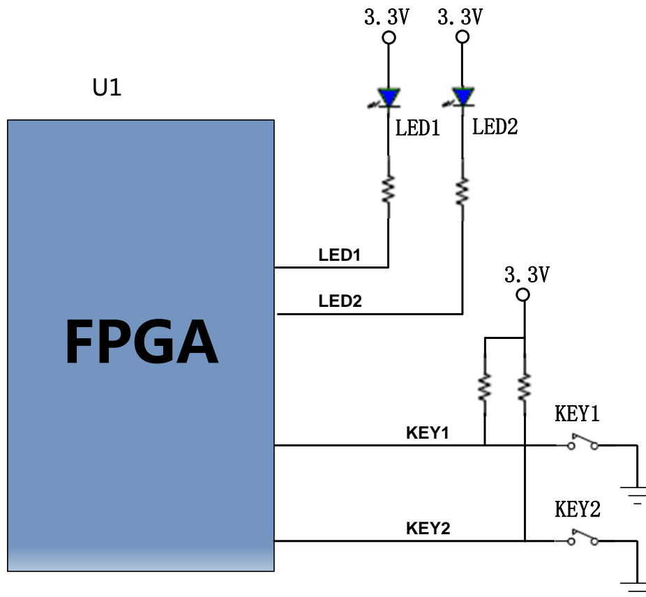
图 3-9-1 用户 LED 灯和按键硬件连接示意图
