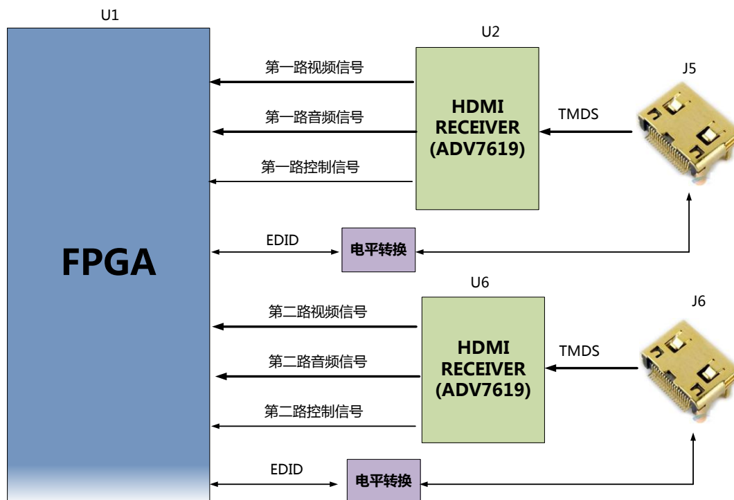
图 3-4-1 HDMI 输入原理图
