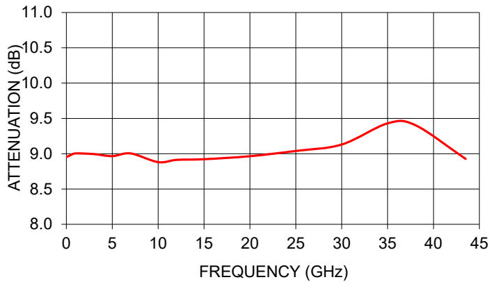
KAT-9+ ATTENUATION
