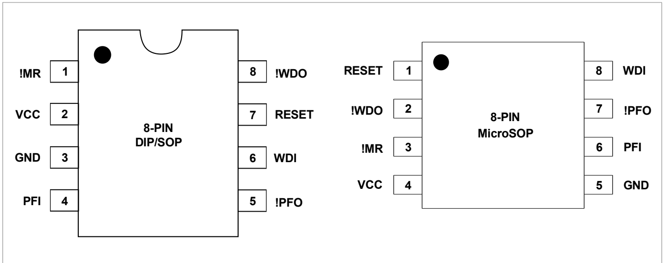
图 2 MAX706P、MAX813L 的管脚分布示意图
