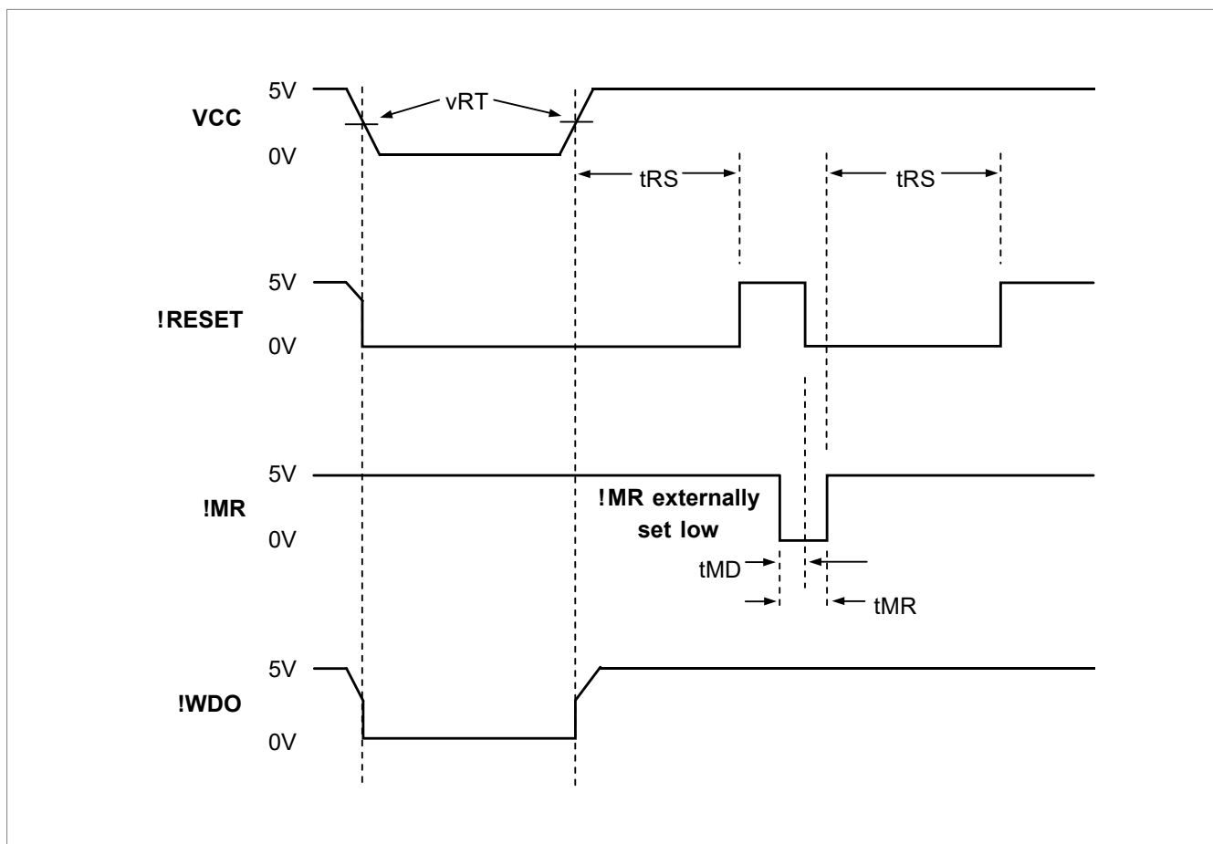
图 5 MAX706P/R/S/T/J, 708R/S/T/J, 705/6/7/8, 813L的复位信号时序图
