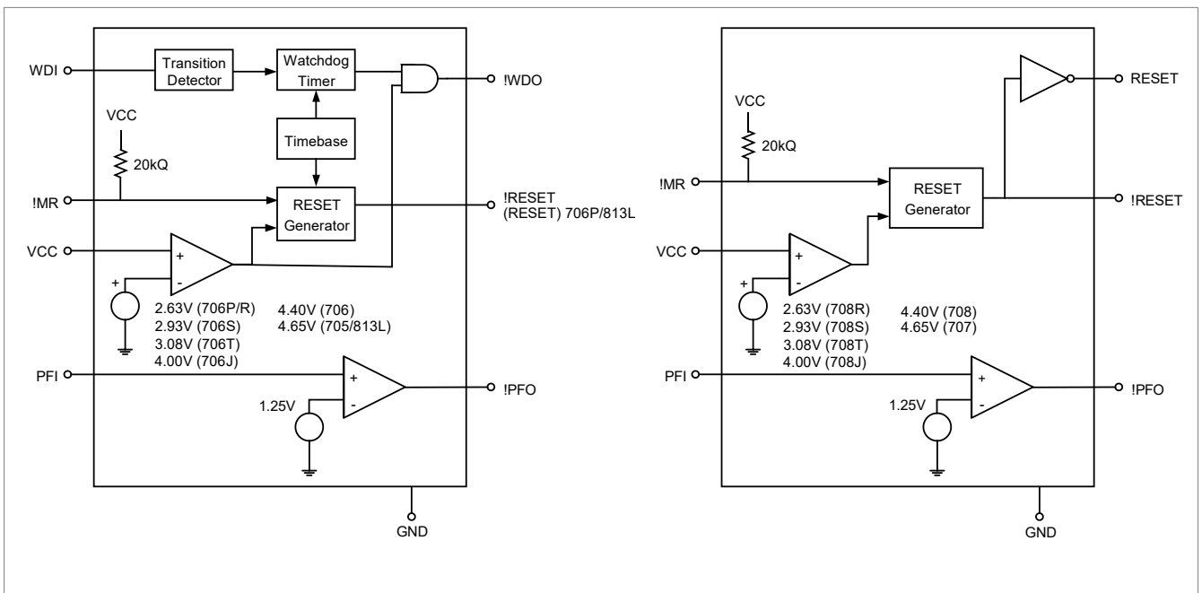
图 1 MAX706P/R/S/T/J, 708R/S/T/J, 705/6/7/8, 的结构示意图
