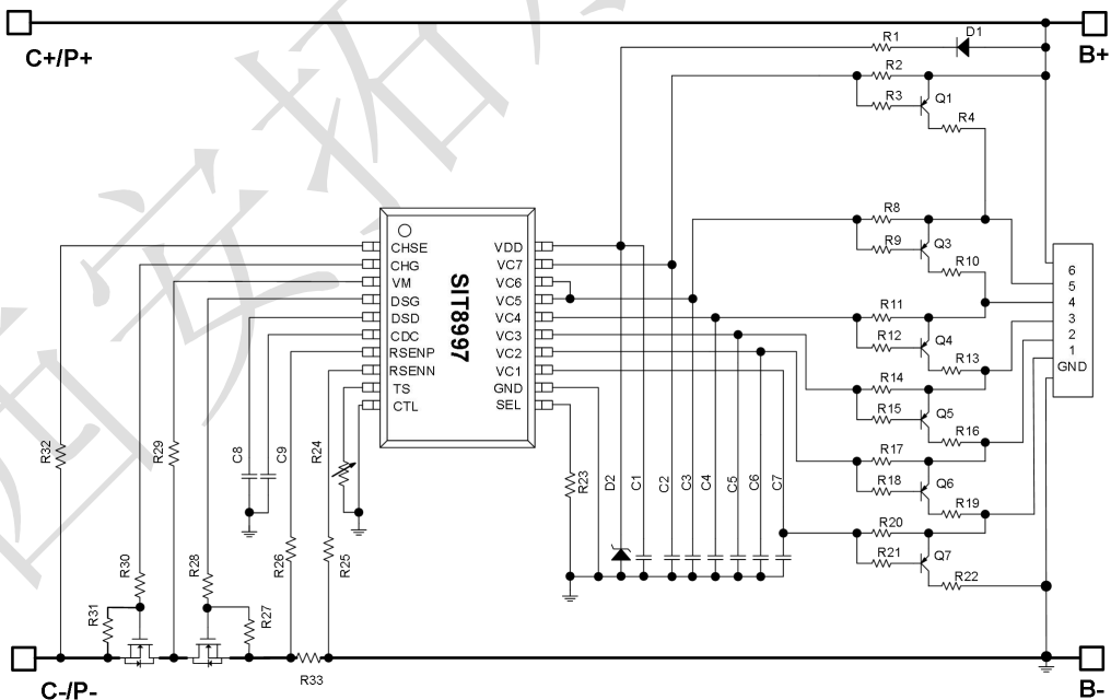
图2 SIT8997典型应用图(6串同口)
