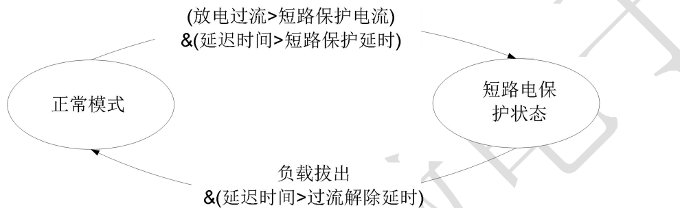
图 8 短路保护状态转移图
