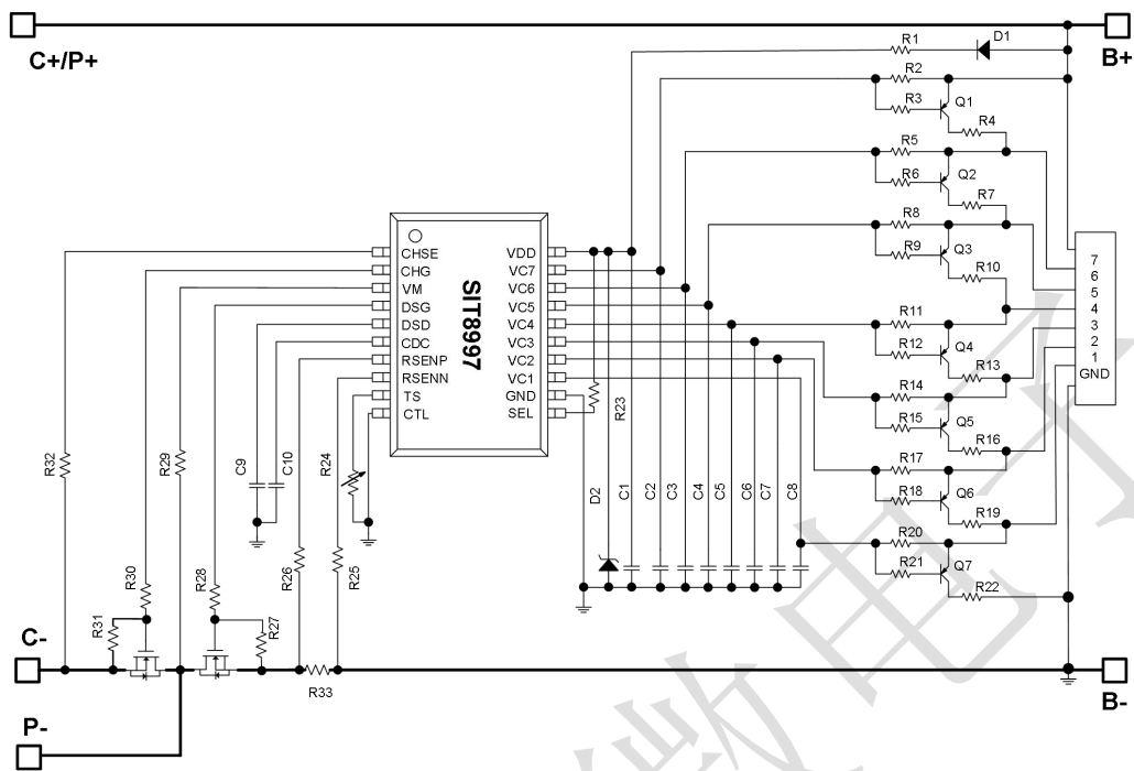
图3 SIT8997典型应用图(7串分口)
