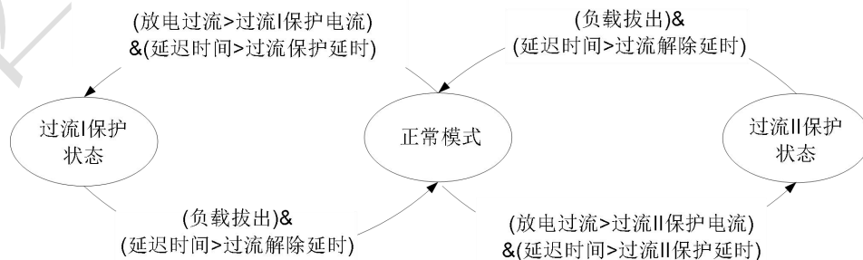
图 7 过流保护状态转移图
