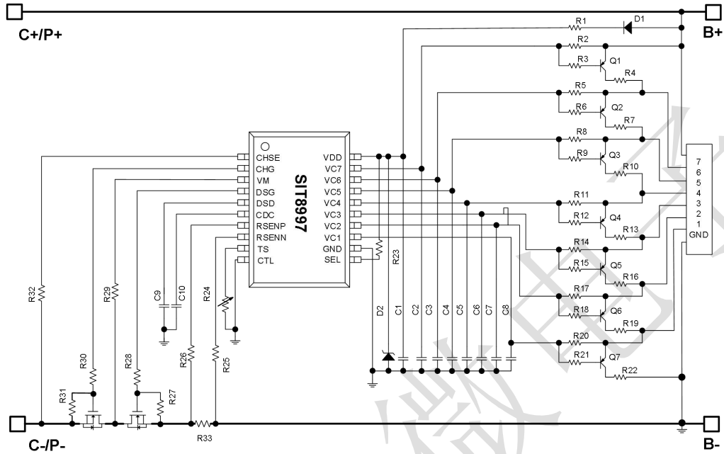
图1 SIT8997典型应用图(7串同口)
