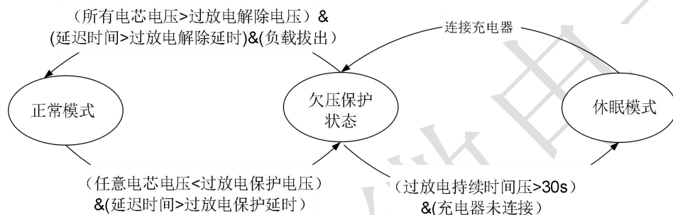
图 6 过放电保护状态转移图
