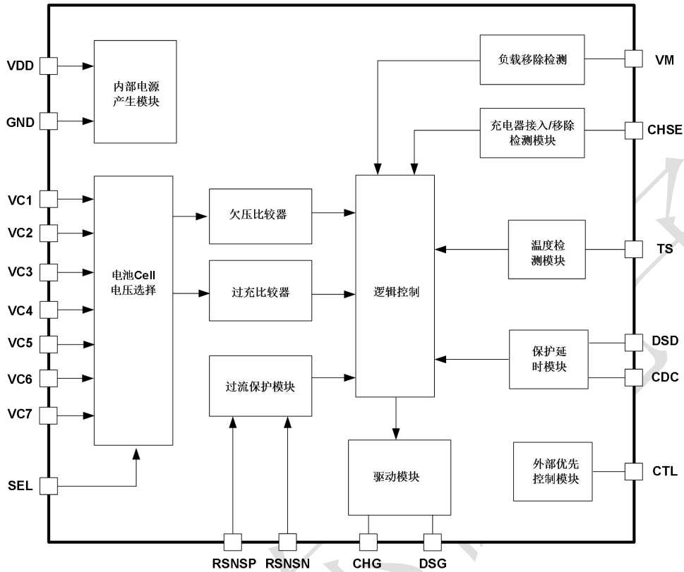
图 4 SIT8997 系统框图
