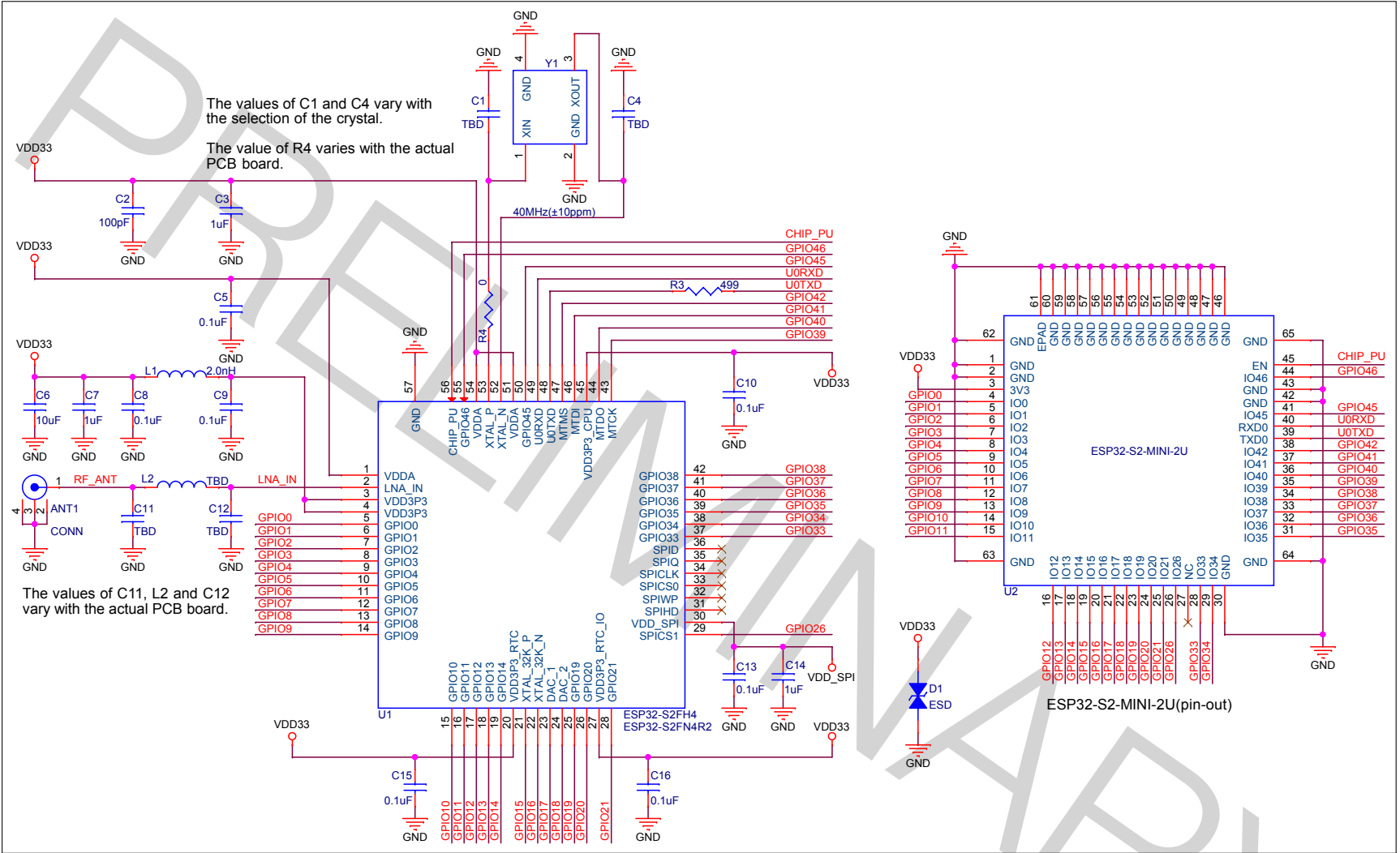
图 6: ESP32-S2-MINI-2U 原理图
