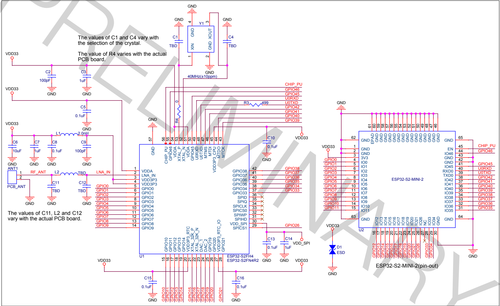
图 5: ESP32-S2-MINI-2 原理图
