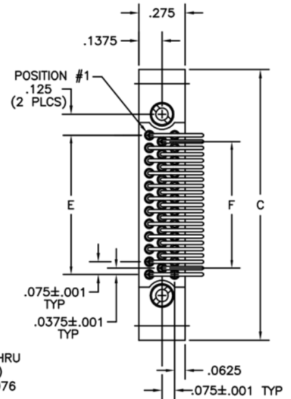
RECEPTACLE
