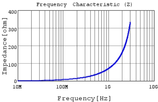
LQP03TN11NH02 |Z|
