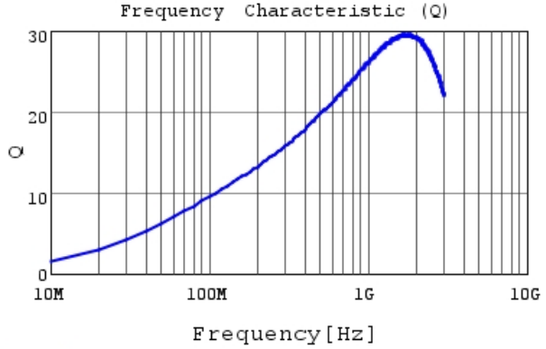
LQP03TN11NH02 Q
