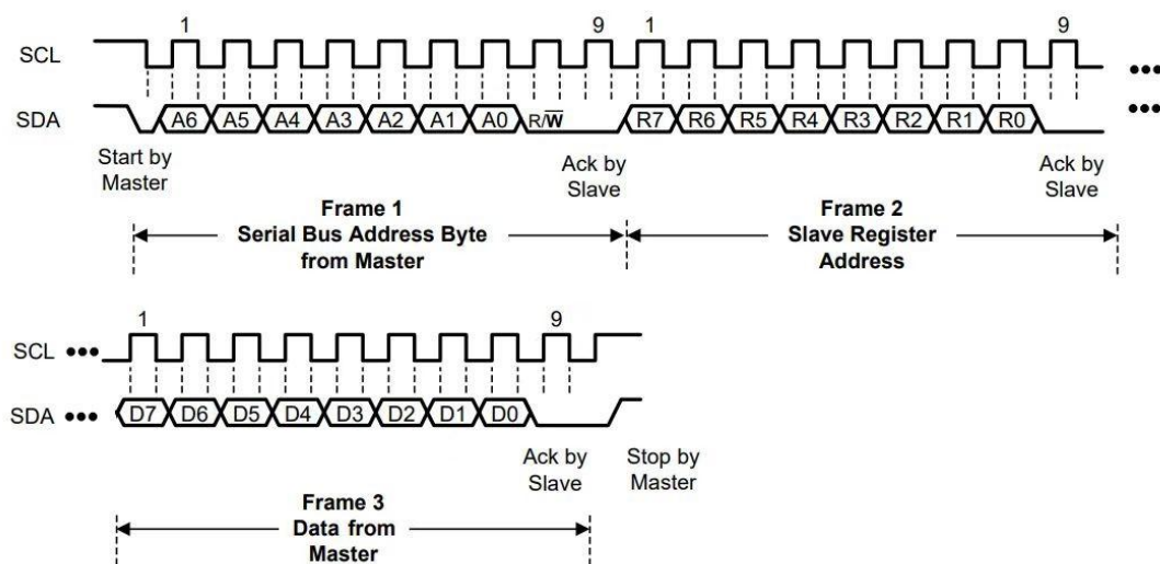
图 7.2-3 I2C 写时序
