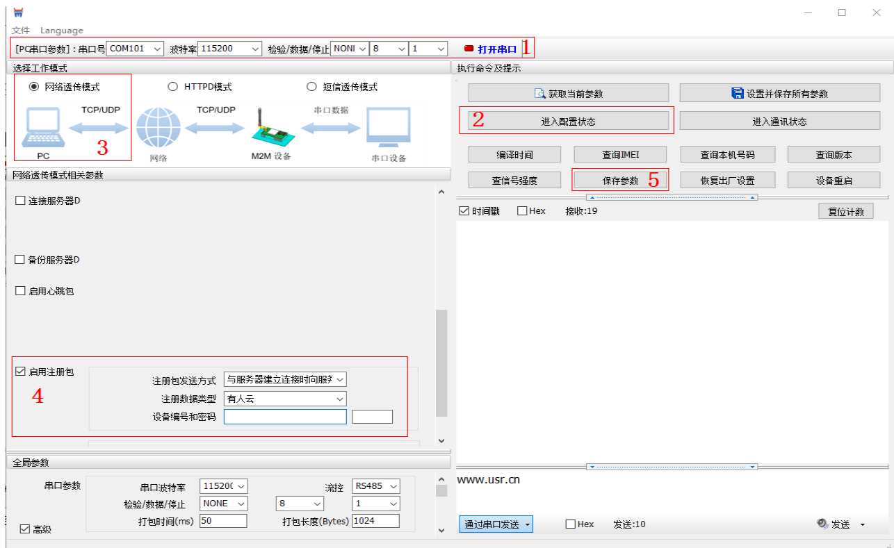
图 20 有人云设置示意图
