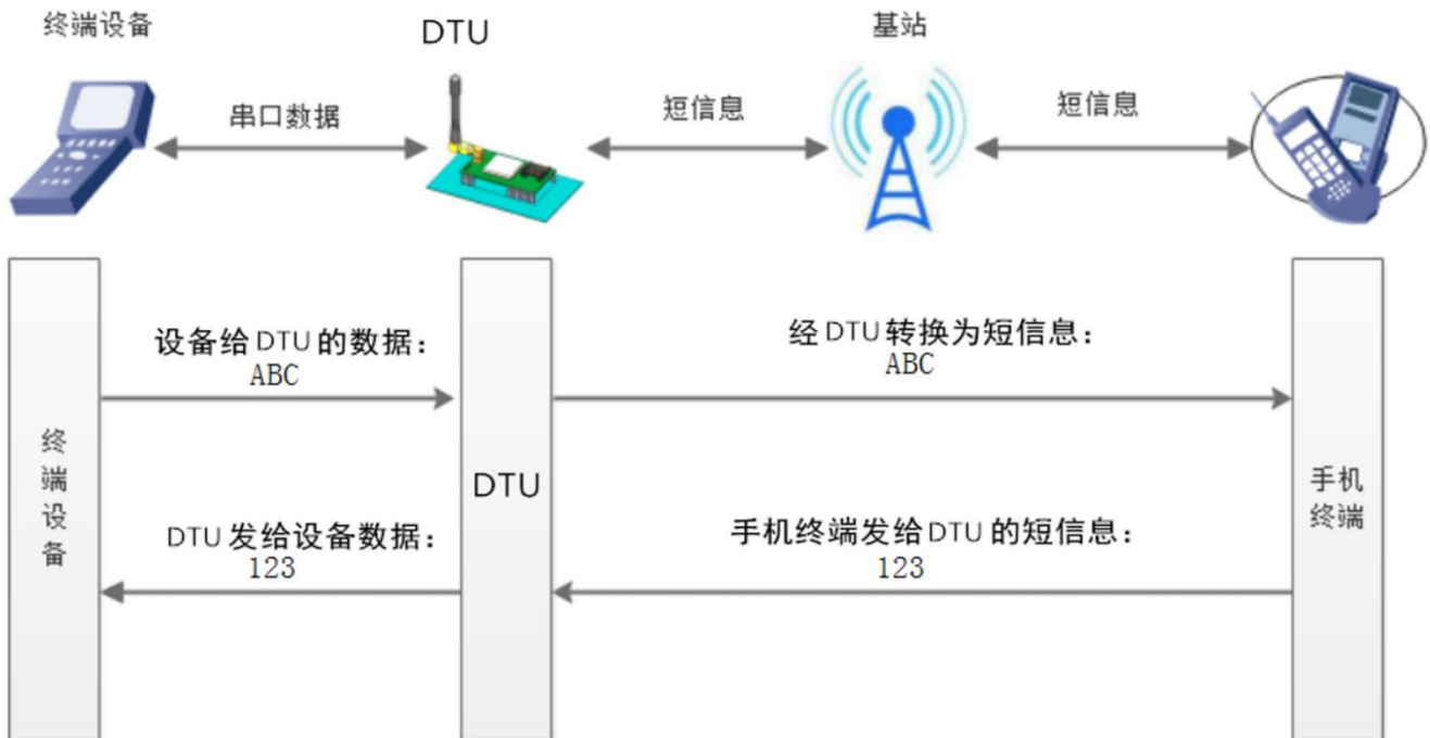
图 12 短信透传模式示意图
