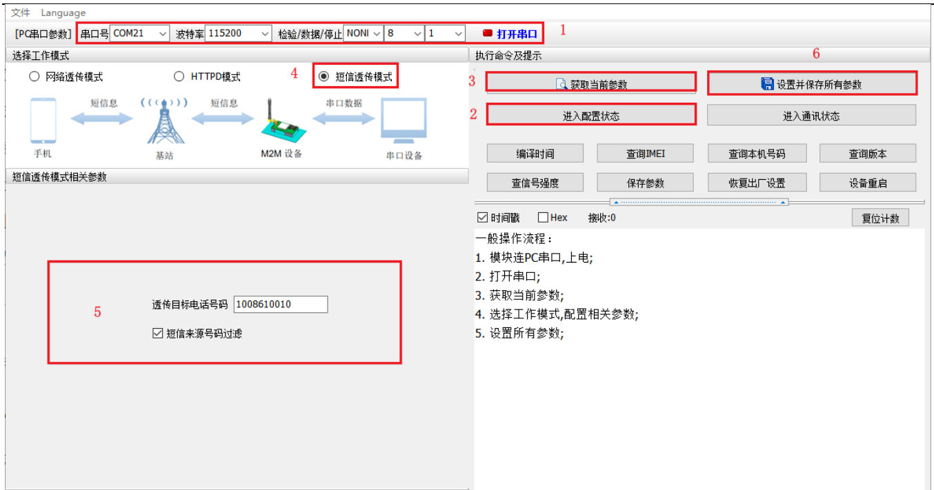
图 13 短信透传模式示意图
