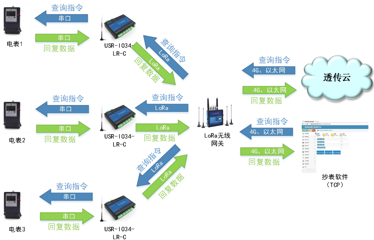
图 32 Modbus 数据采集系统示意图
