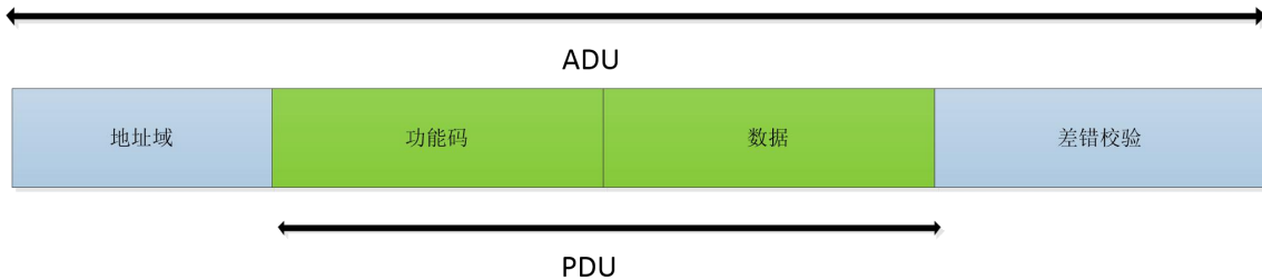
图 34 Modbus RTU 帧
