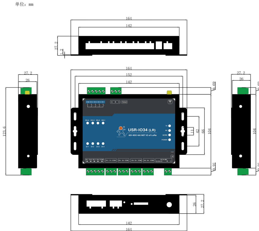
图 24 USR-IO34-LR-C 尺寸图
