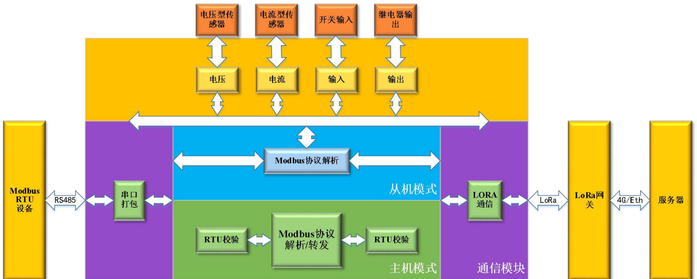
USR-IO34-LR-C 功能框图
