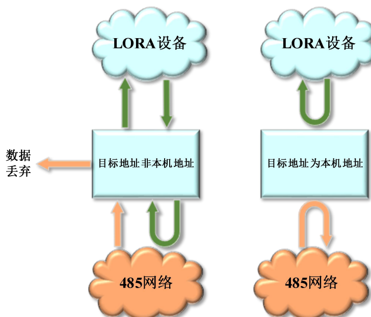
图 27 主机模式数据流向图
