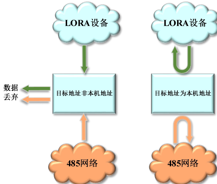
图 28 从机模式数据流向图
