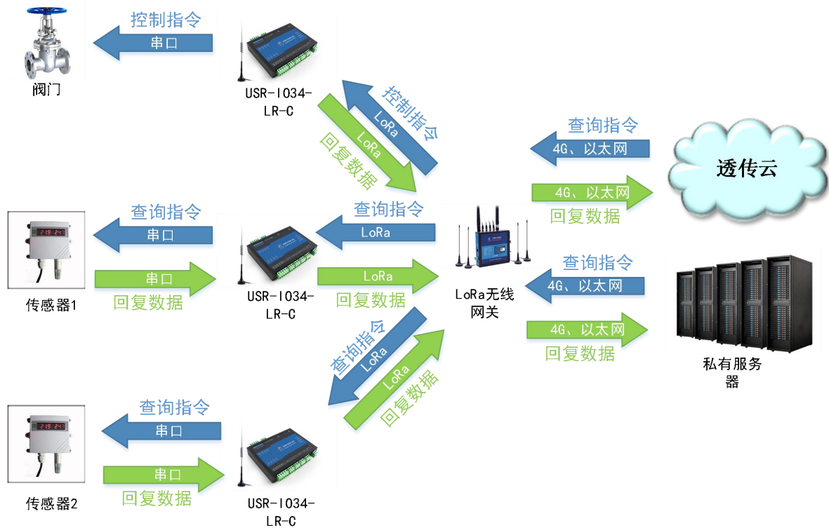
图 33 定点数据采集及控制系统示意图
