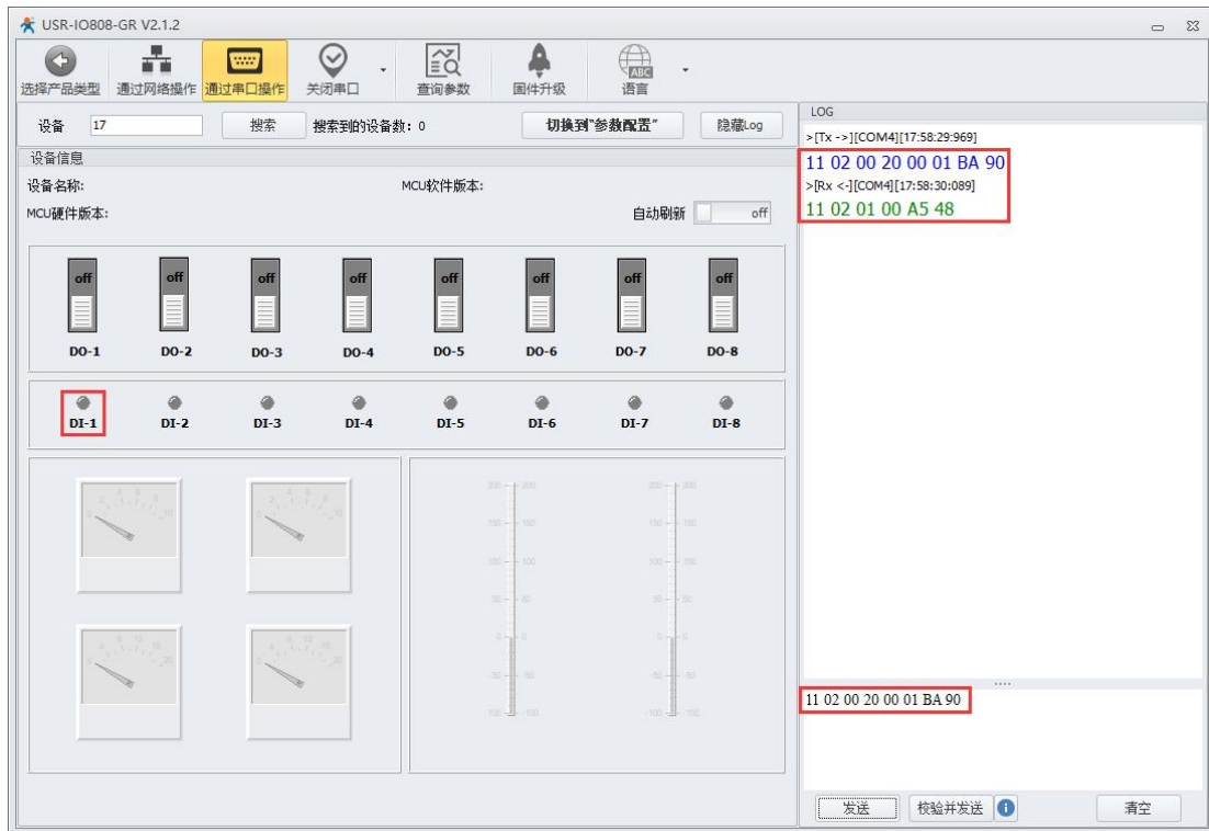
图 16 电平检测
