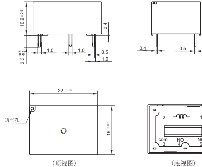
外形图
