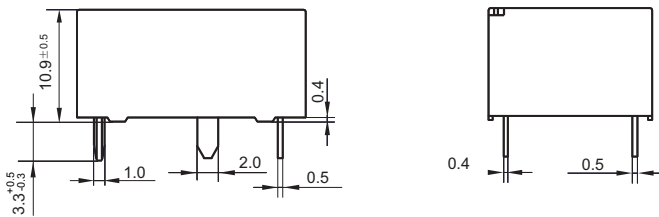
外形图
