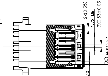
剖面: B-B
