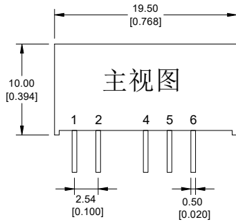
封装尺寸图
