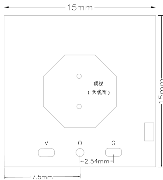
图 4.2 MW10G15-B 模块尺寸图
