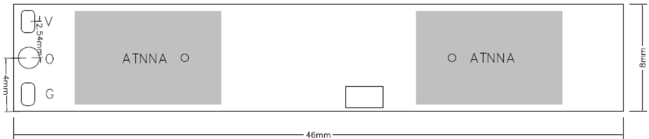
图 4.2 MW5S10-C 模块尺寸图
