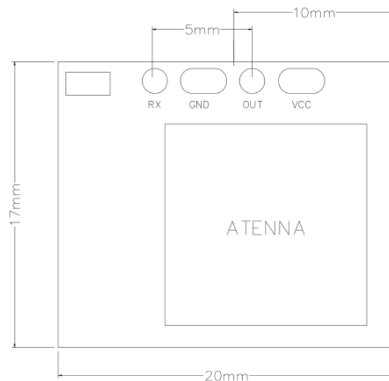
图 4.2 MW5S20-B 模块尺寸图
