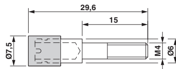
尺寸图
