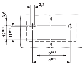
钻孔图
