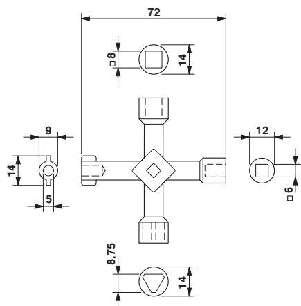
尺寸图
