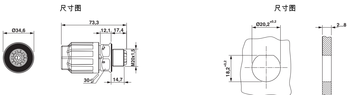
QPD W 5x2,5 M20尺寸图
