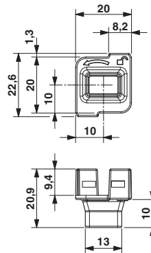
尺寸图
