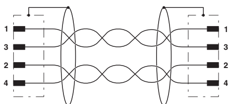
电路图
