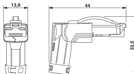
RJ45 连接器，IP20，弯头
