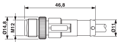
针式，M12 x 1，直头，屏蔽
