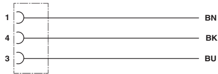
电路图
