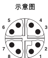
M12针式连接器引脚分配, 8芯, 插头侧视图
